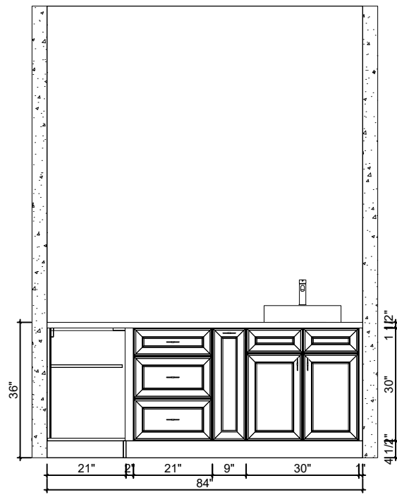
1-A Elevation(1/3"=1'-0")
