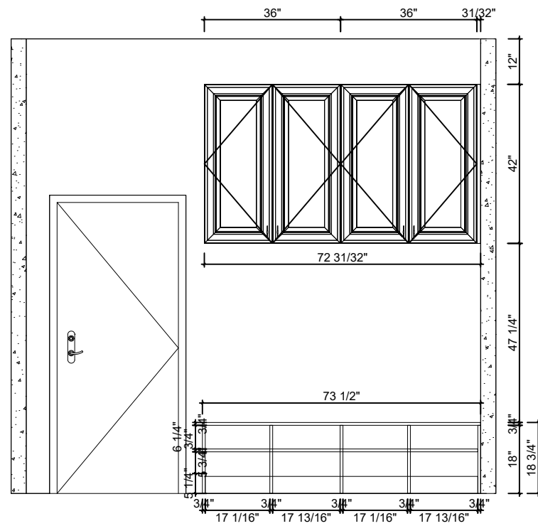
1-A Elevation(1/3"=1'-0")
