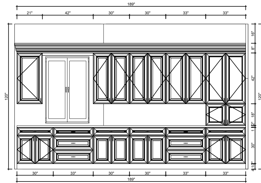
1-A Elevation(1/4"=1'-0")
